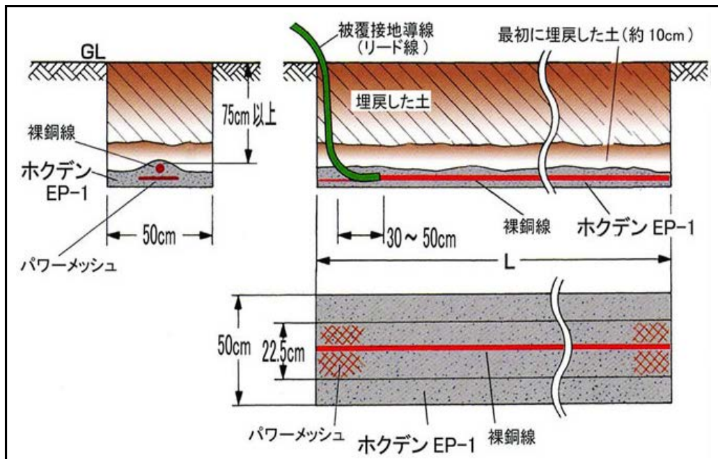
図1. 帯状電極施工図
